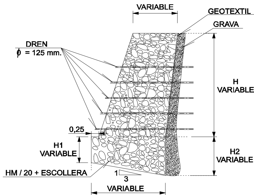
SECCIÓN TIPO DE MURO
