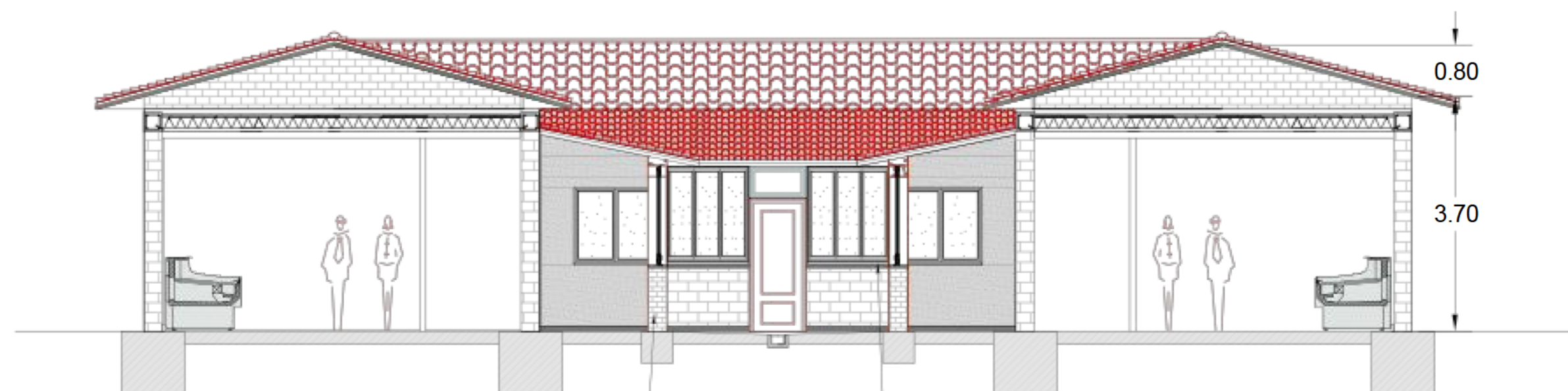
SECCION B-B'
