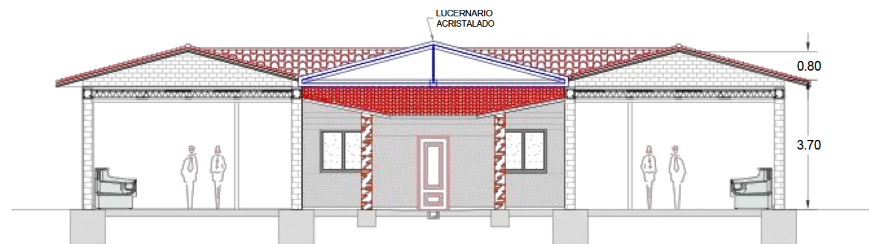
SECCION A-A'
