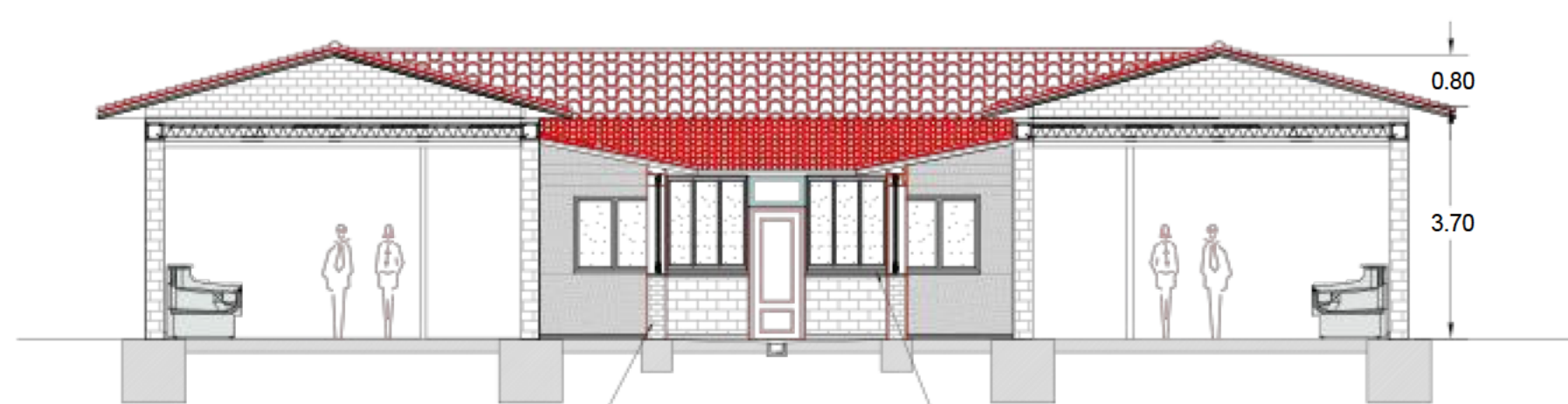
SECCION B-B'
