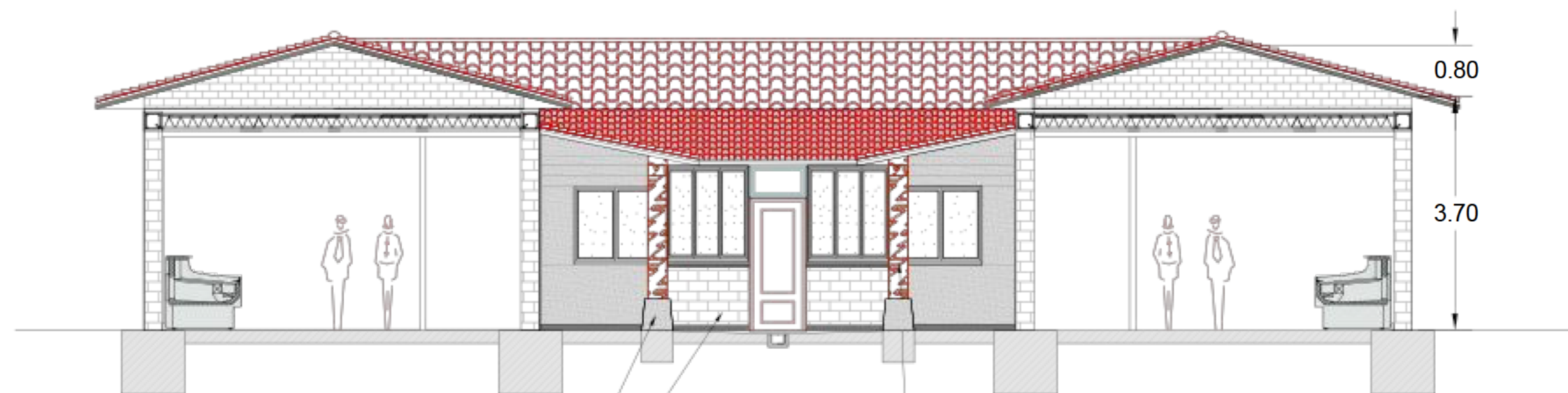
SECCION A-A'
